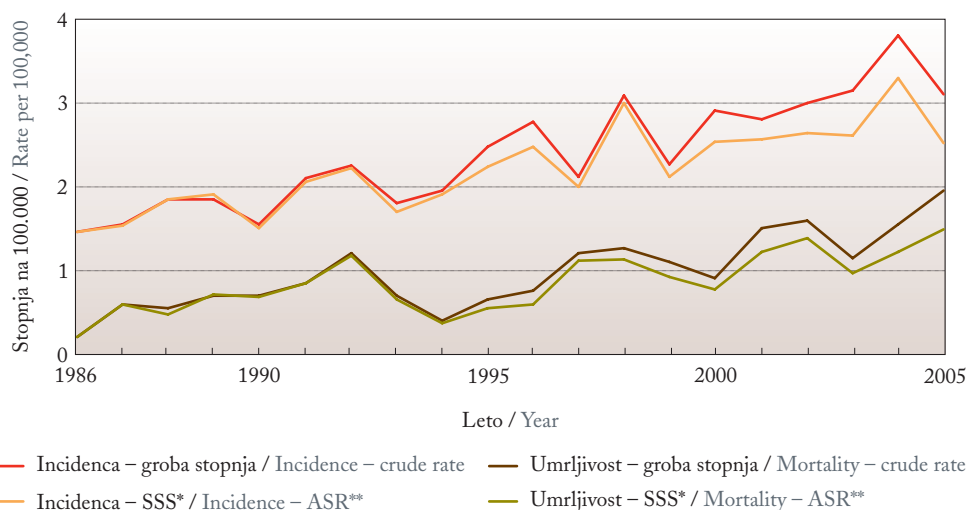
Slika 1: Groba in starostno standardizirana incidenčna in umrljivostna stopnja raka mehkih tkiv, Slovenija 1986–2005.
