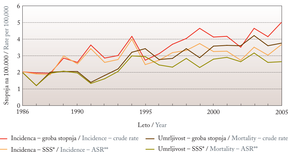
Slika 1: Groba in starostno standardizirana incidenčna in umrljivostna stopnja plazmocitoma, Slovenija 1986–2005.
